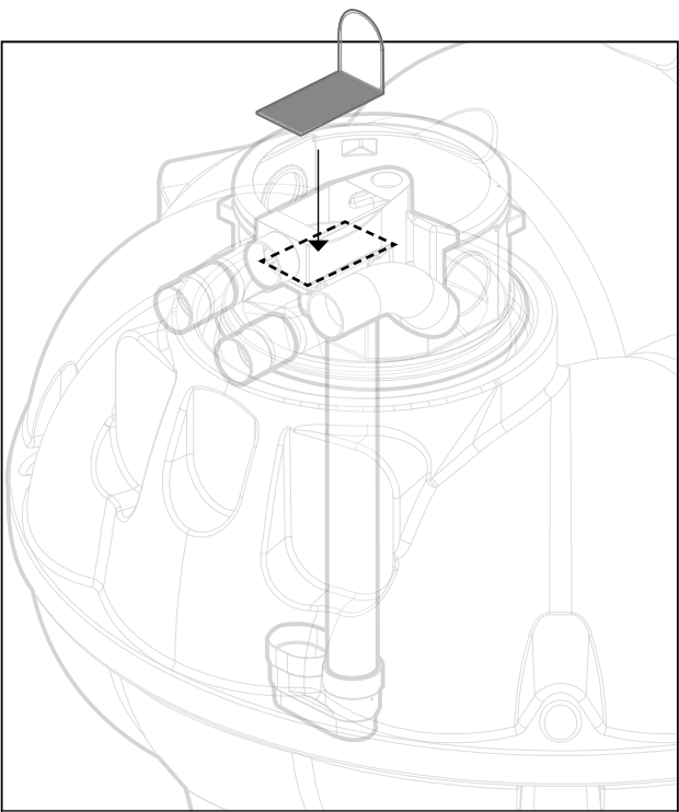
Incliner la grille de filtration pour l'introduire dans le corps de filtration
