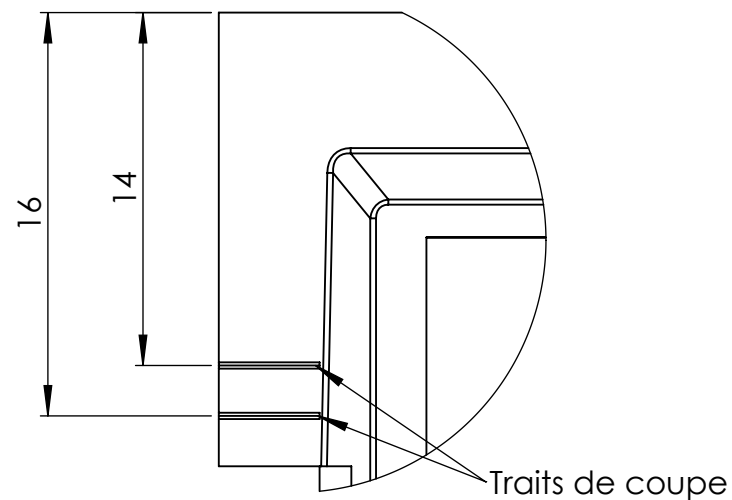
DÉTAIL B
