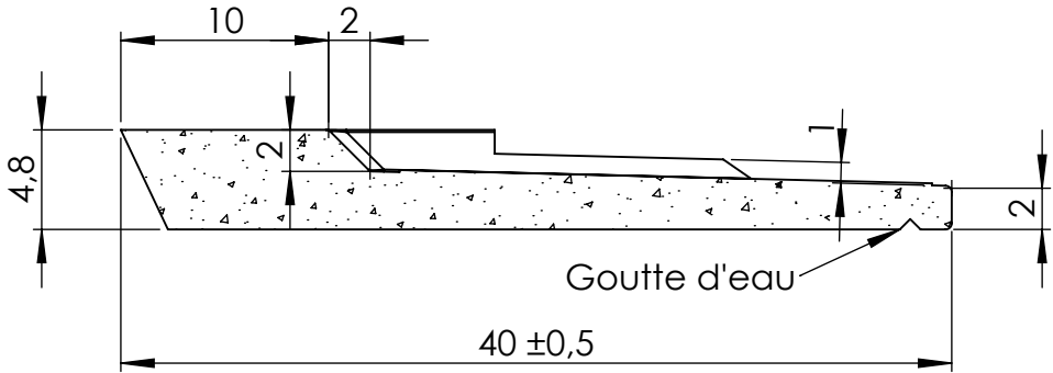
COUPE A-A Seuil de baie
