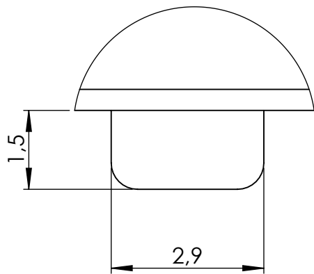
DÉTAIL A ÉCARTEURS
