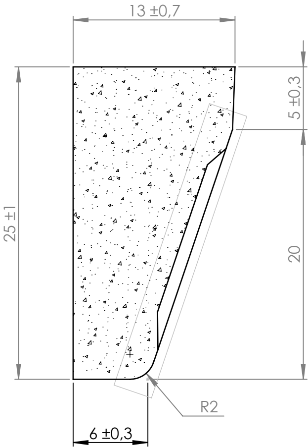
COUPE A-A
