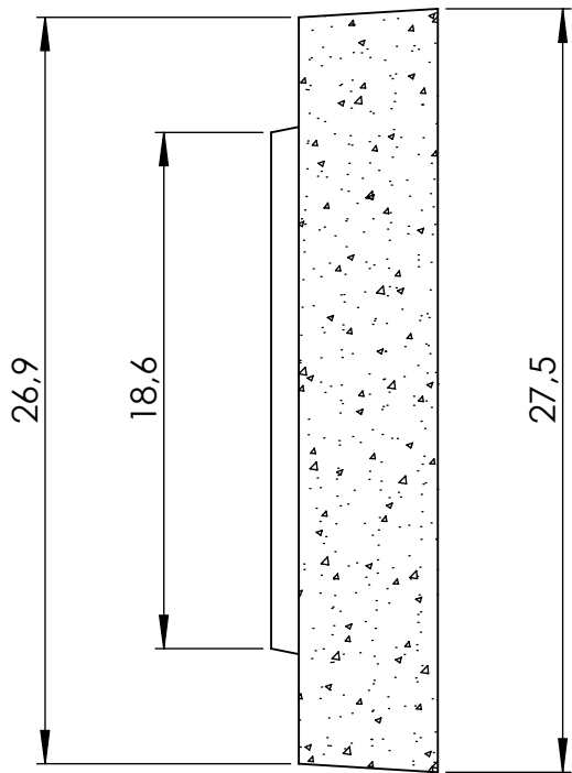
COUPE A-A
