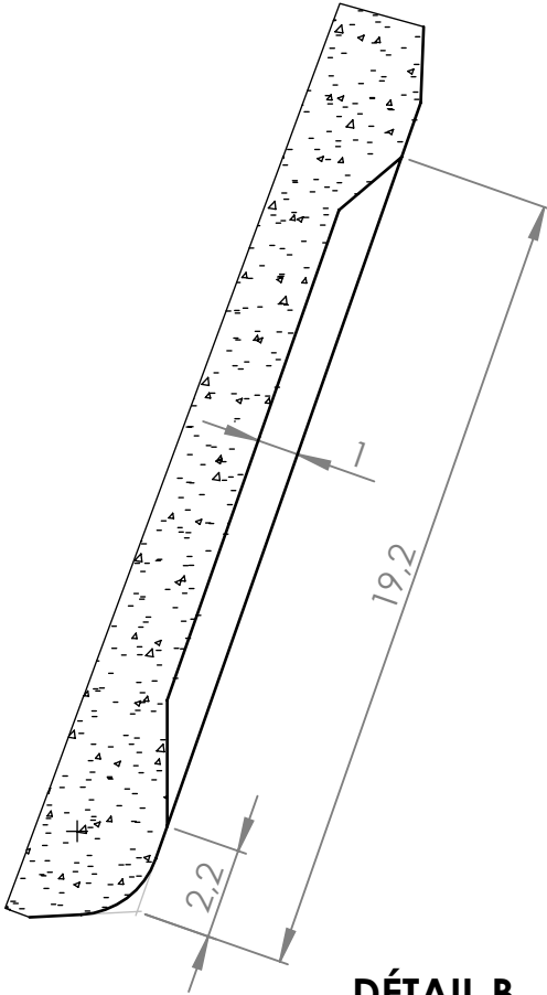
DÉTAIL B
