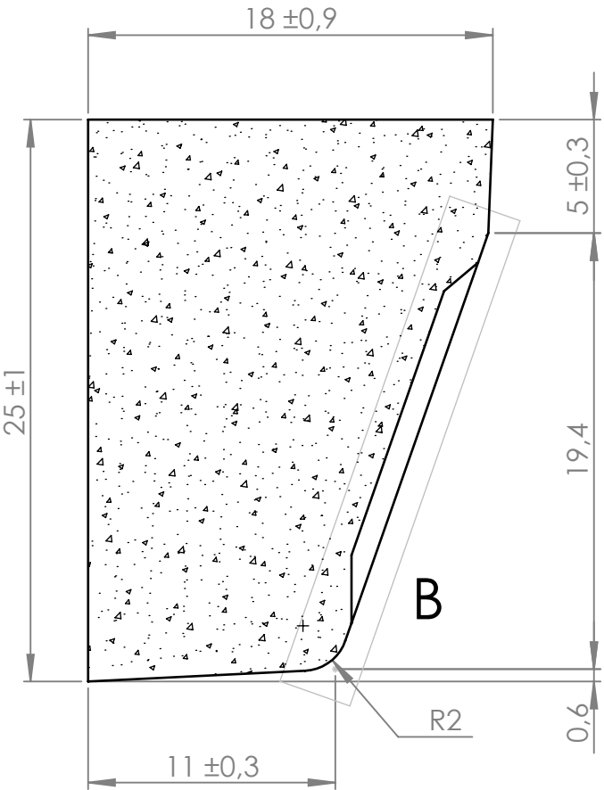
COUPE A-A
