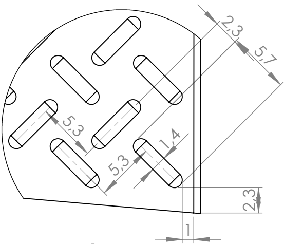
DÉTAIL A
