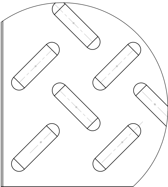
DÉTAIL A
