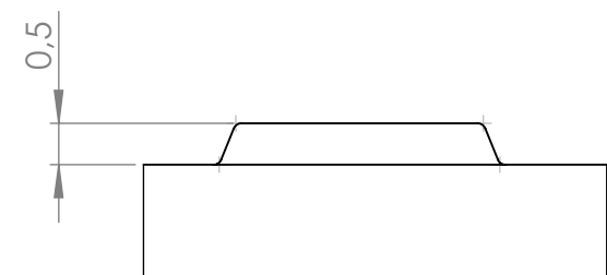
DÉTAIL A : détails nervures
