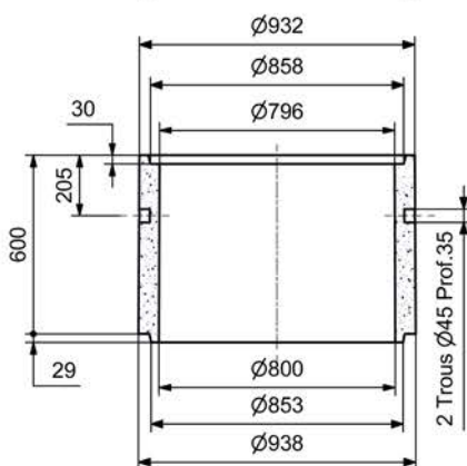
BUSE DE PUITS A EMBOITEMENTS Ø Int. 0,80 m Ht. 0,60 m PLEINE
