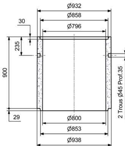
BUSE DE PUITS A EMBOITEMENTS Ø Int. 0,80 m Ht. 0,90 m PLEINE
